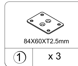
Angle Bracket Abrazadera Équerre TSF2620
